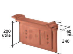
Rive universelle (3 au ml) Réf. 1050
