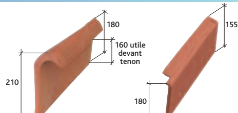
Rive individuelle gauche à recouvrement (3,9 au ml) Réf. 220.42
