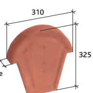
Fronton pour faîtière 1/2 ronde à recouvrement Réf. 807
