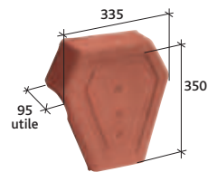
Fronton de rive universelle Réf. 1080
